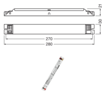
Caractéristiques Osram LED Driver OPTOTRONIC 55/220-240/1A0 CS L G2
